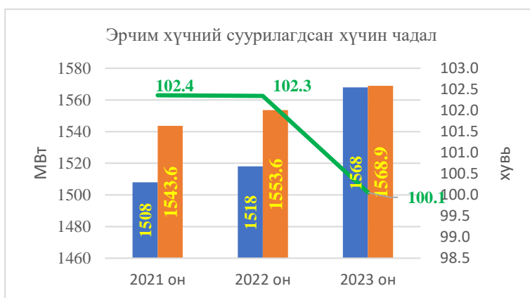
Дүрслэл 15. Эрчим хүчний суурилагдсан хүчин чадал
